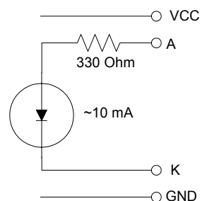
Fig. 4.1 – Interlock diagram
