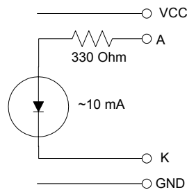
Fig. 4.1 – Interlock diagram
