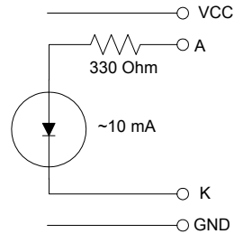
Fig. 4.1 – Interlock diagram
